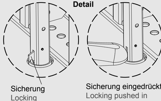
Geländer absenken/anheben Lower/lift railing
