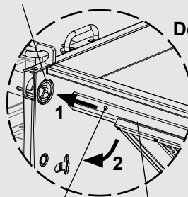
Sicherheitsaufnahme Safety lock
