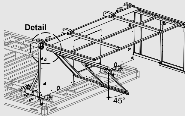
Seitengeländeraufnahme Connection point for side rail
