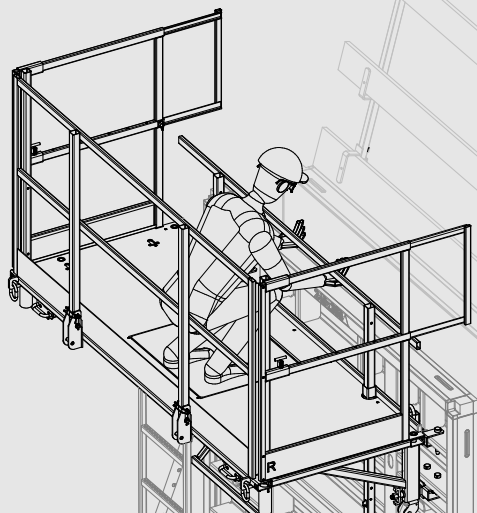
Geländer absenken/anheben Lower/lift railing
