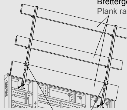
PROTECTO Fußbretthalter PROTECTO toe board retainer
