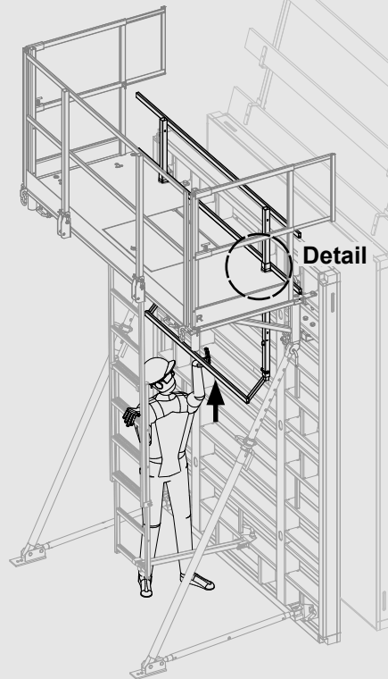
Vorlaufgeländer anheben Lift advancing guardrail
